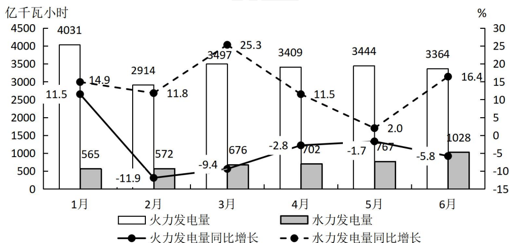
2015 年 1—6 月我国火力、水力发电量及其增长情况
