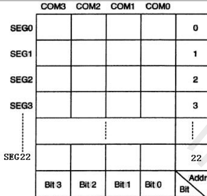
RAM 映象图
