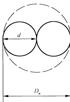
图 1 1\times 2 结构钢绞线外形示意图
