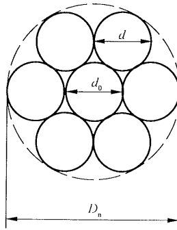
图 3 1×7 结构钢绞线外形示意图
