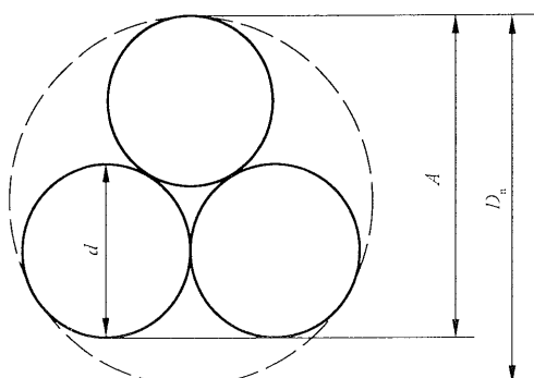
图 2 1\times 3 结构钢绞线外形示意图
