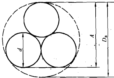
图 2 1×3 结构钢绞线外形示意图
