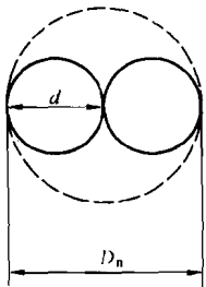
图 1 1×2 结构钢绞线外形示意图
