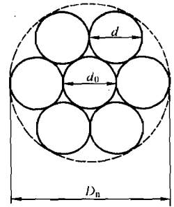
图 3 1×7 结构钢绞线外形示意图
