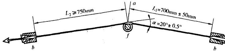
图 B.1 偏斜拉伸试验装置
