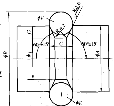
图 B.2 心轴
