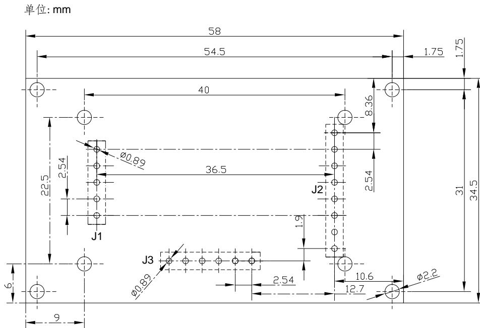
图 1 TX523LT 封装
