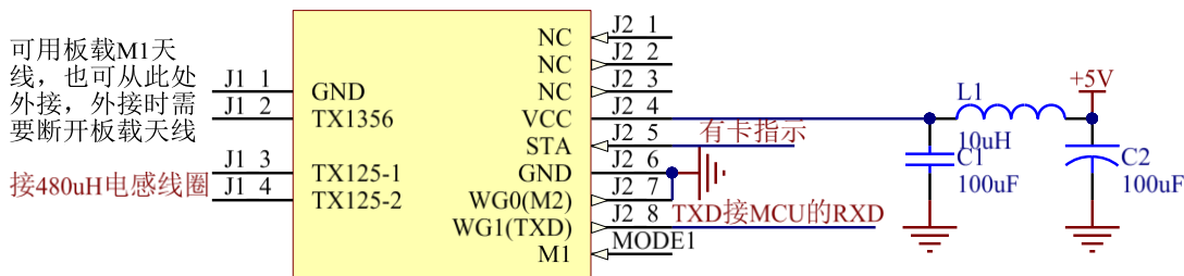
图 3.1 TX601T 串口通信 (9600, N, 1)
