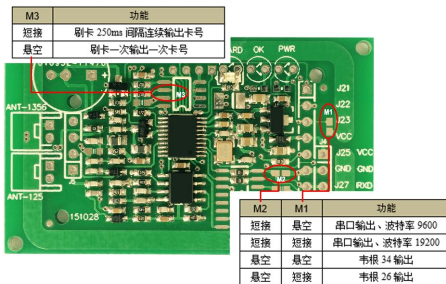
图 2.1 TX601 工作模式设置图解
