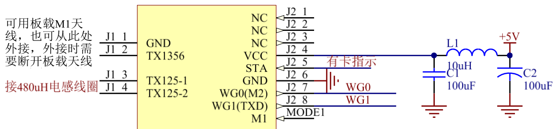
图 3.2 TX601T 韦根 34 接口
