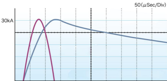
放电波形图
