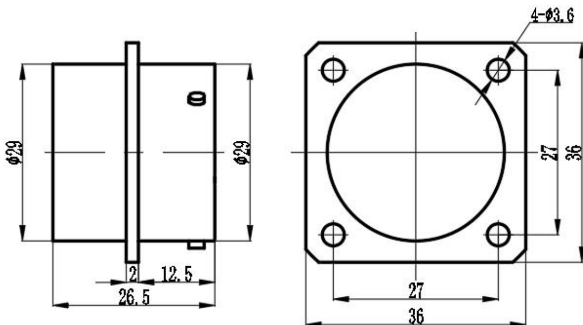
插座外形图（Y50X-1832ZJ10）
