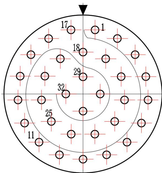
型谱（从插针的插合面看绝缘板）
