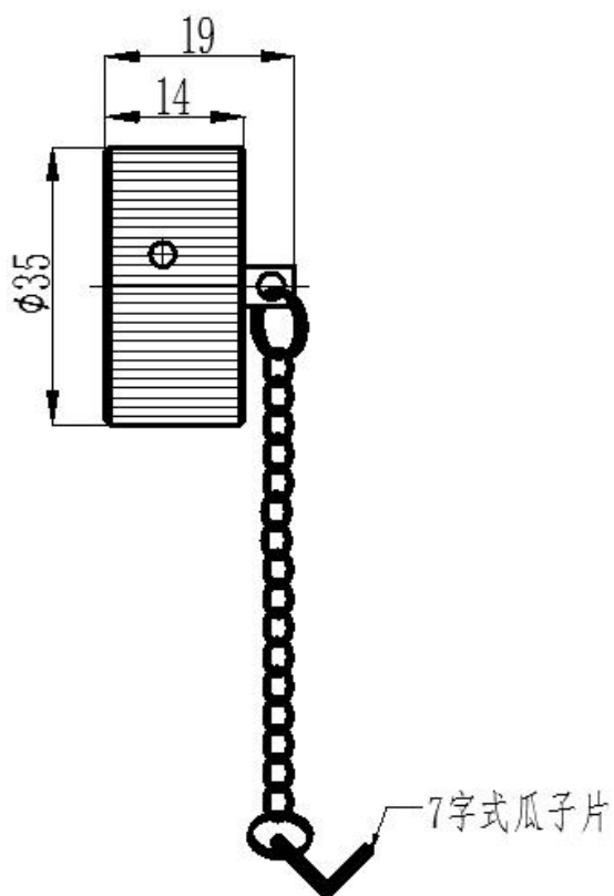
防尘盖外形图
