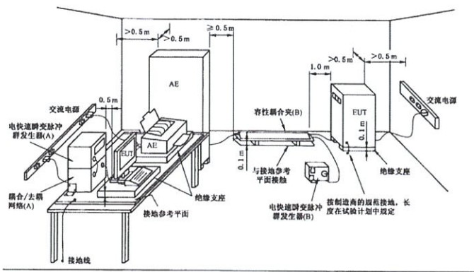
布置图
