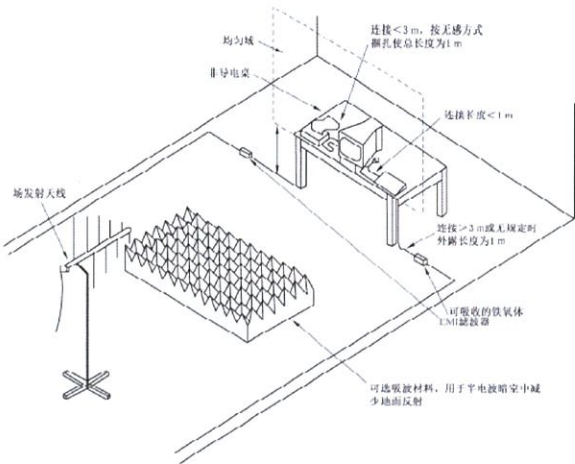
布置图
