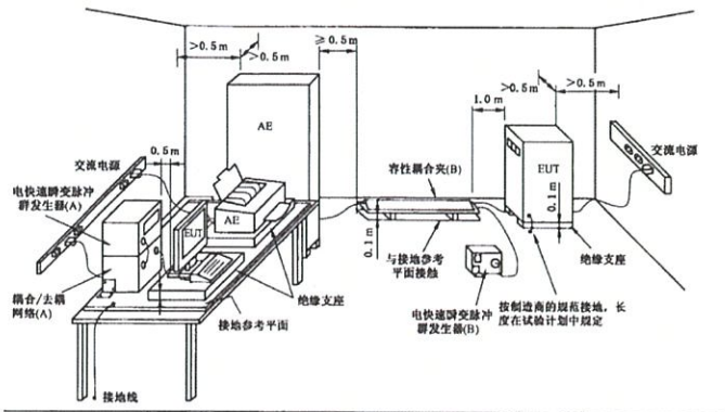
布置图
