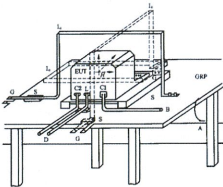
布置图
