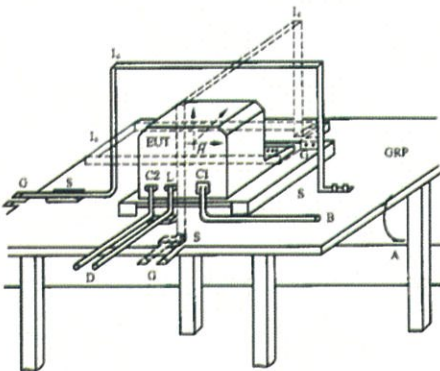
布置图
