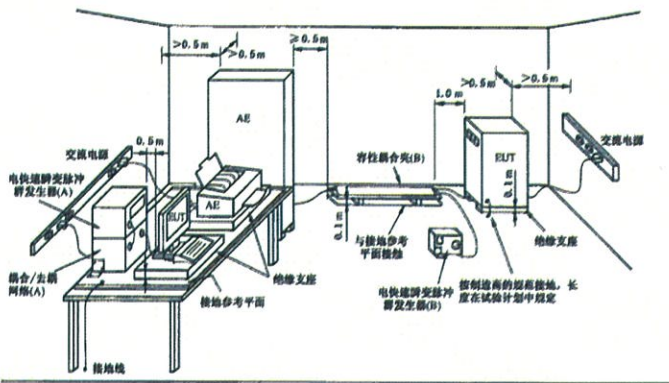
布置图
