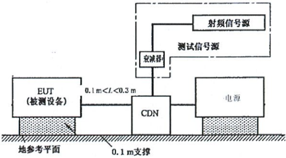
布置图
