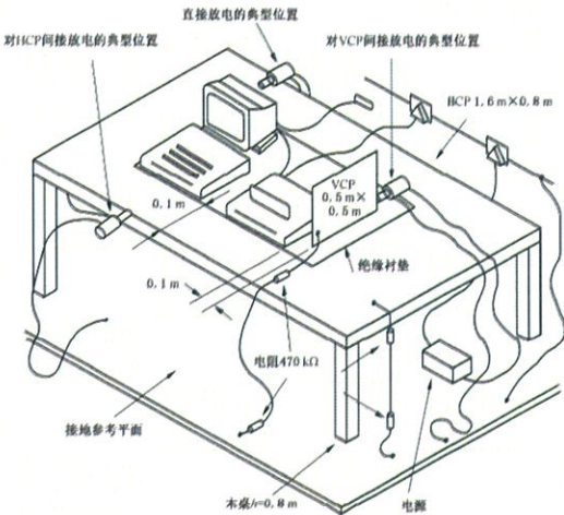
布置图
