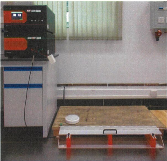
布置照片
