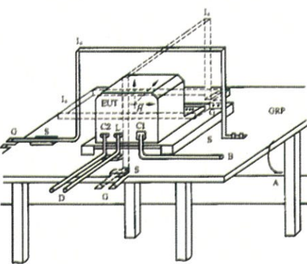
布置图
